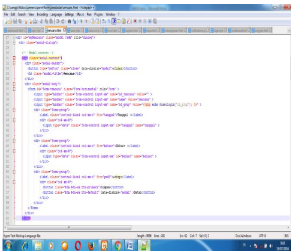
Gambar 12. Source Code Halaman Tambah Rencana
