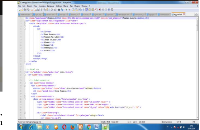
Gambar 14. Source Code Halaman Tambah Anggota
